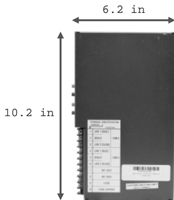
Left Side
