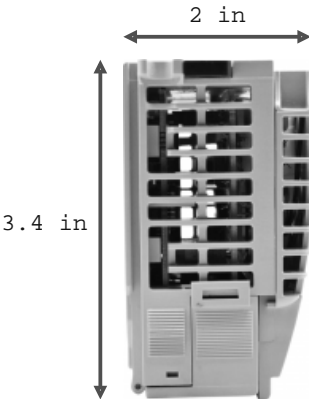
Bottom
